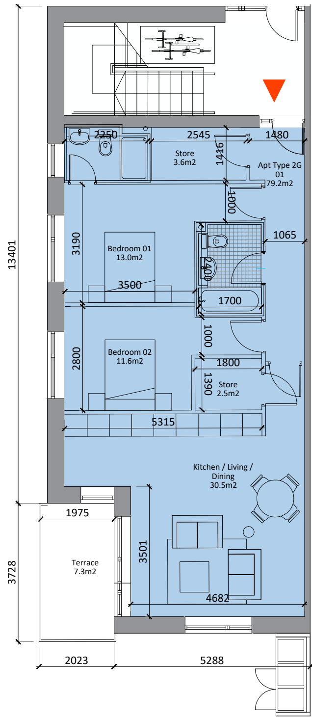
Level 01 1:100
